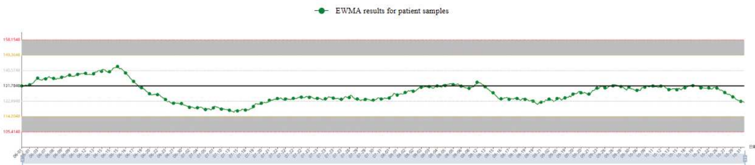
DXI800 TT4 82.15-200.19 EWMA chart (Tradition-PBRTQC \lambda : 0.02)
